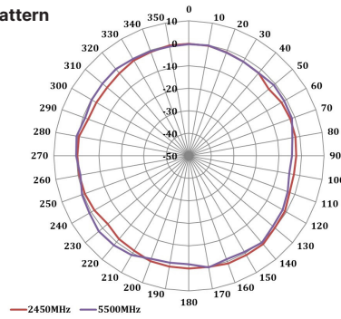
H-Plane Pattern
