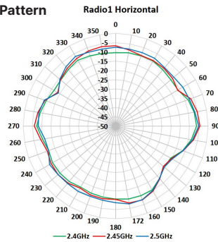
H-Plane Pattern
