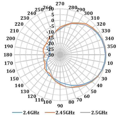
Radio1 - Vertical
