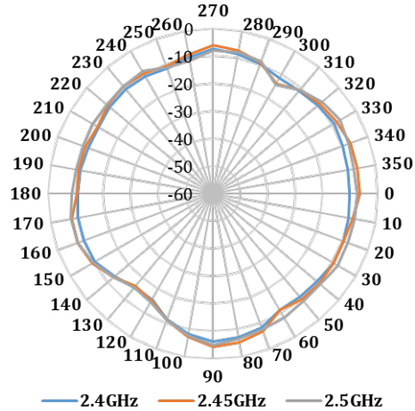
Radio1 - Horizontal
