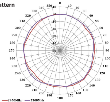
H-Plane Pattern
