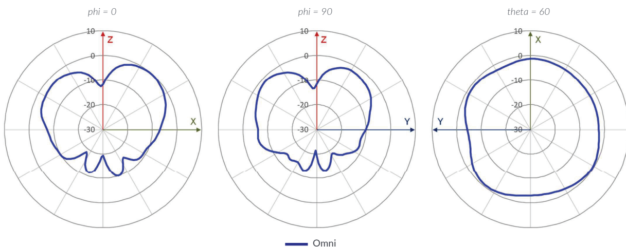
2.4 Ghz Omni BLE @ 2440MHz
