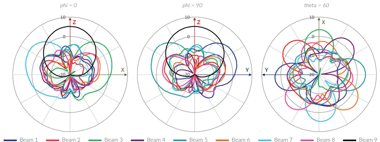
2.4 Ghz Directional BLE @ 2480MHz
