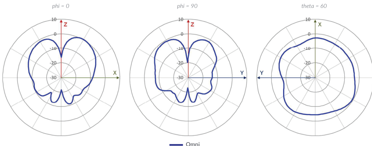
2.4 Ghz Omni BLE @ 2480MHz
