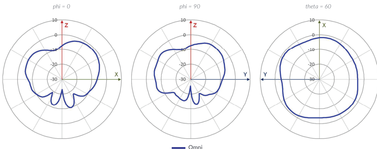
2.4 Ghz Omni BLE @ 2400MHz
